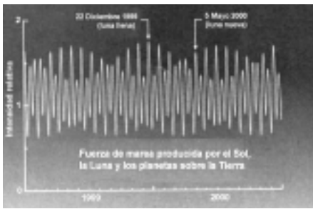
GRÁFICA QUE MUESTRA LA INTENSIDAD DE LA FUERZA DE MAREA PRODUCIDA POR EL SOL, LA LUNA Y TODOS LOS PLANETAS DEL SISTEMA SOLAR SOBRE LA TIERRA EN EL PERÍODO 1999-2000.
