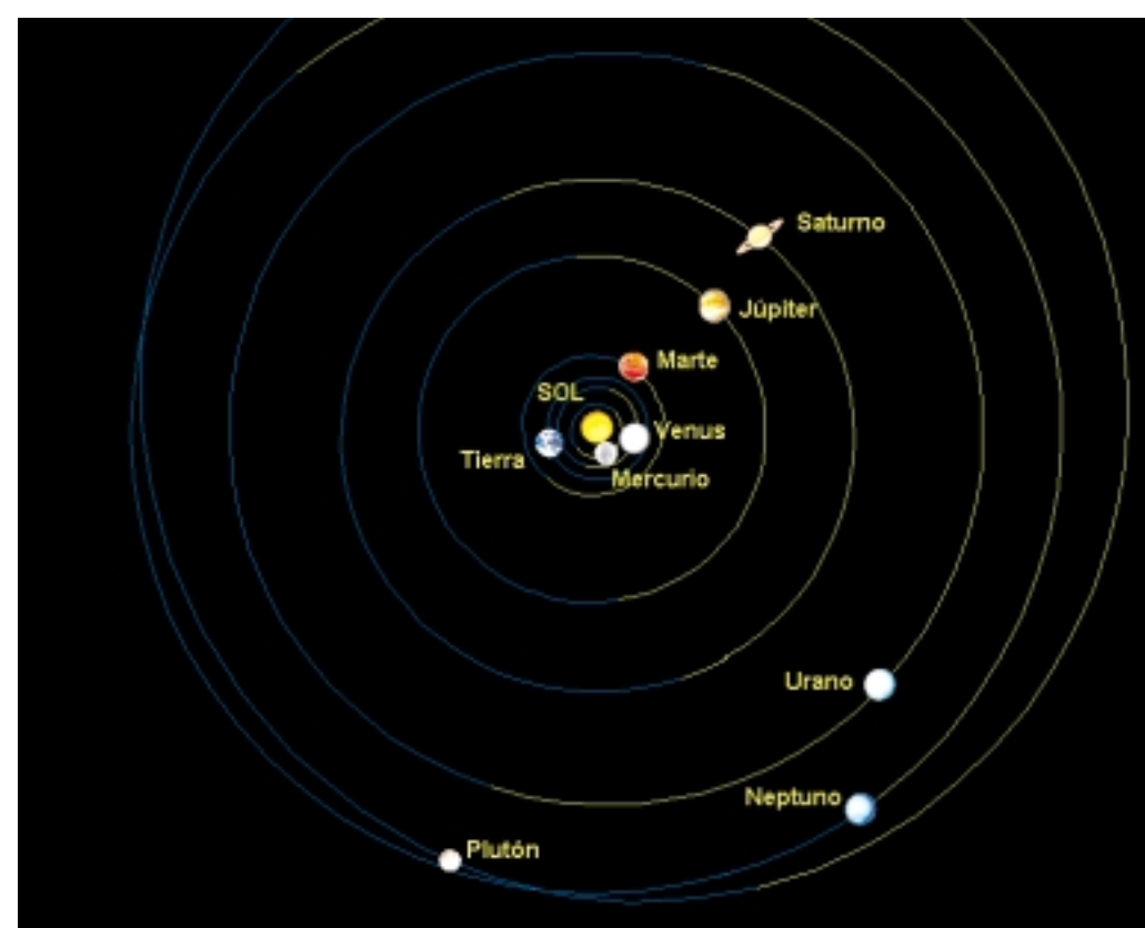
POSICIÓN RELATIVA DE LOS PLANETAS DEL SISTEMA SOLAR EL 5 DE MAYO DE 2000. NÓTESE QUE LA AGRUPACIÓN SE PRODUCE AL LADO OPUESTO DEL SOL, EN RELACIÓN CON LA TIERRA.
